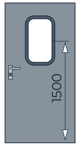
Oblò 400x700 FM L min=800
