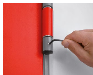
Cerniera portante dotata di viti per la registrazione verticale a sfere reggispinta
