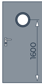
Oblò Ø300 FM L min=700
