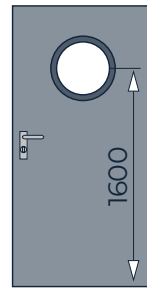
Oblò Ø400 FM L min=800
