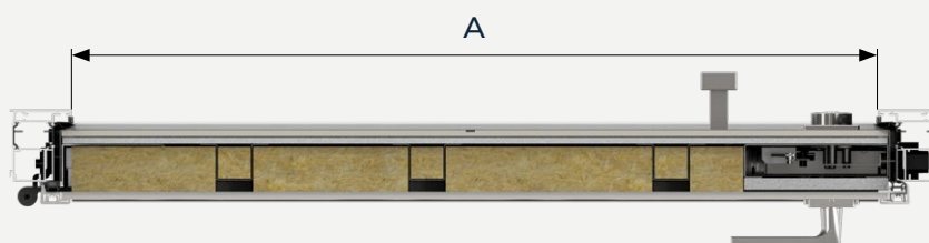
Sezione orizzontale
